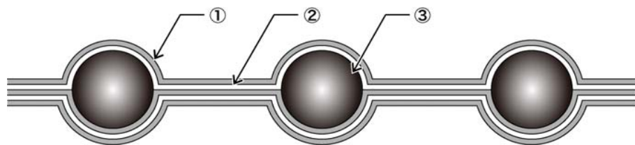
断面図
